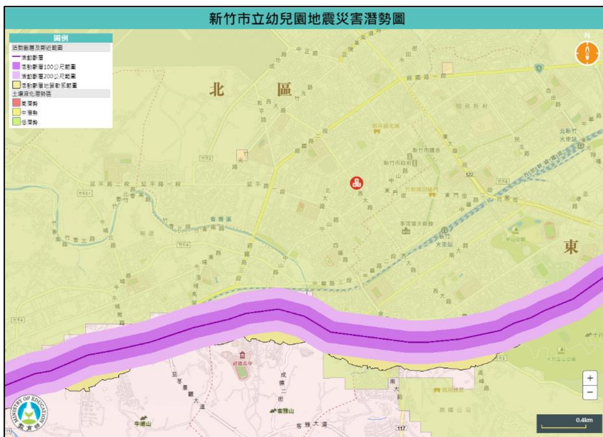
圖 2.4.1 地震災害潛勢圖（參考） （瀏覽日期：109 年 4 月 15 日）
