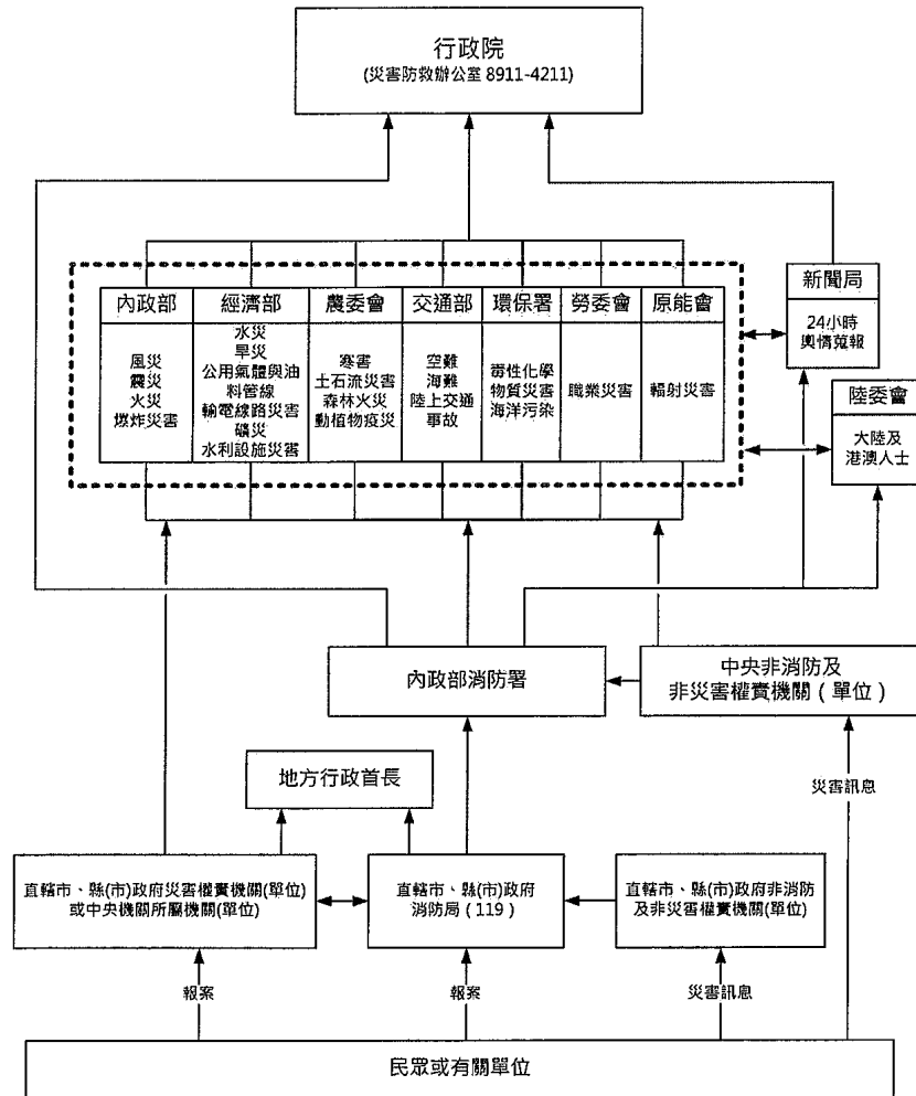
災害緊急通報系統圖
